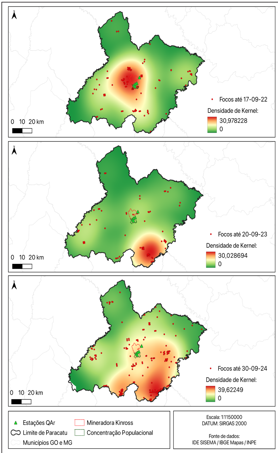
Figura 22. Estações de monitoramento QAr, estimador de Kernel e focos de incêndio.
