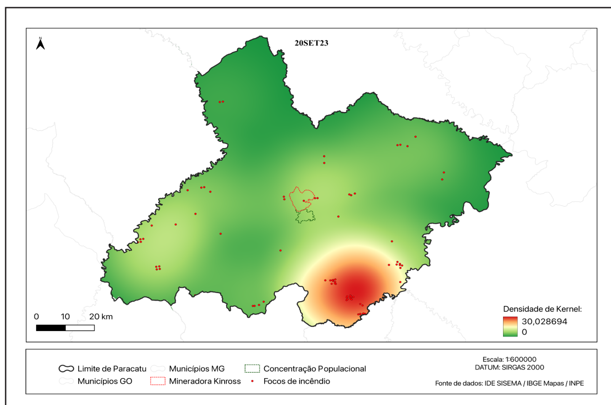
Figura 18. Estimador de Kernel para os focos de incêndio até 20SET23
