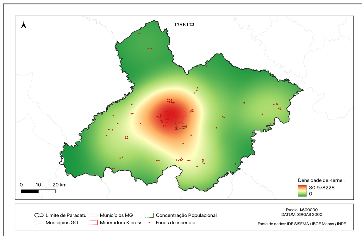
Figura 16. Estimador de Kernel para os focos de incêndio até 17SET22
