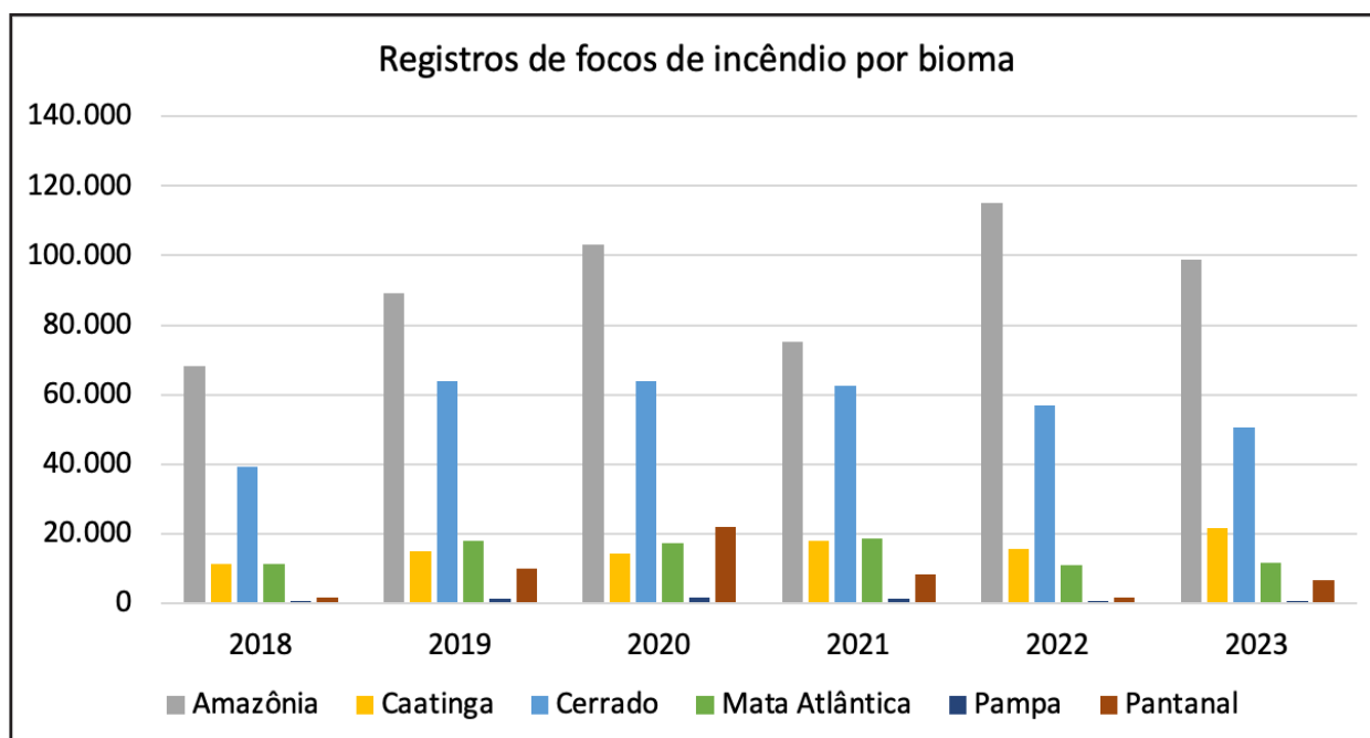
Figura 2. Número de focos de incêndio nos biomas brasileiros de 2018 a 2023
