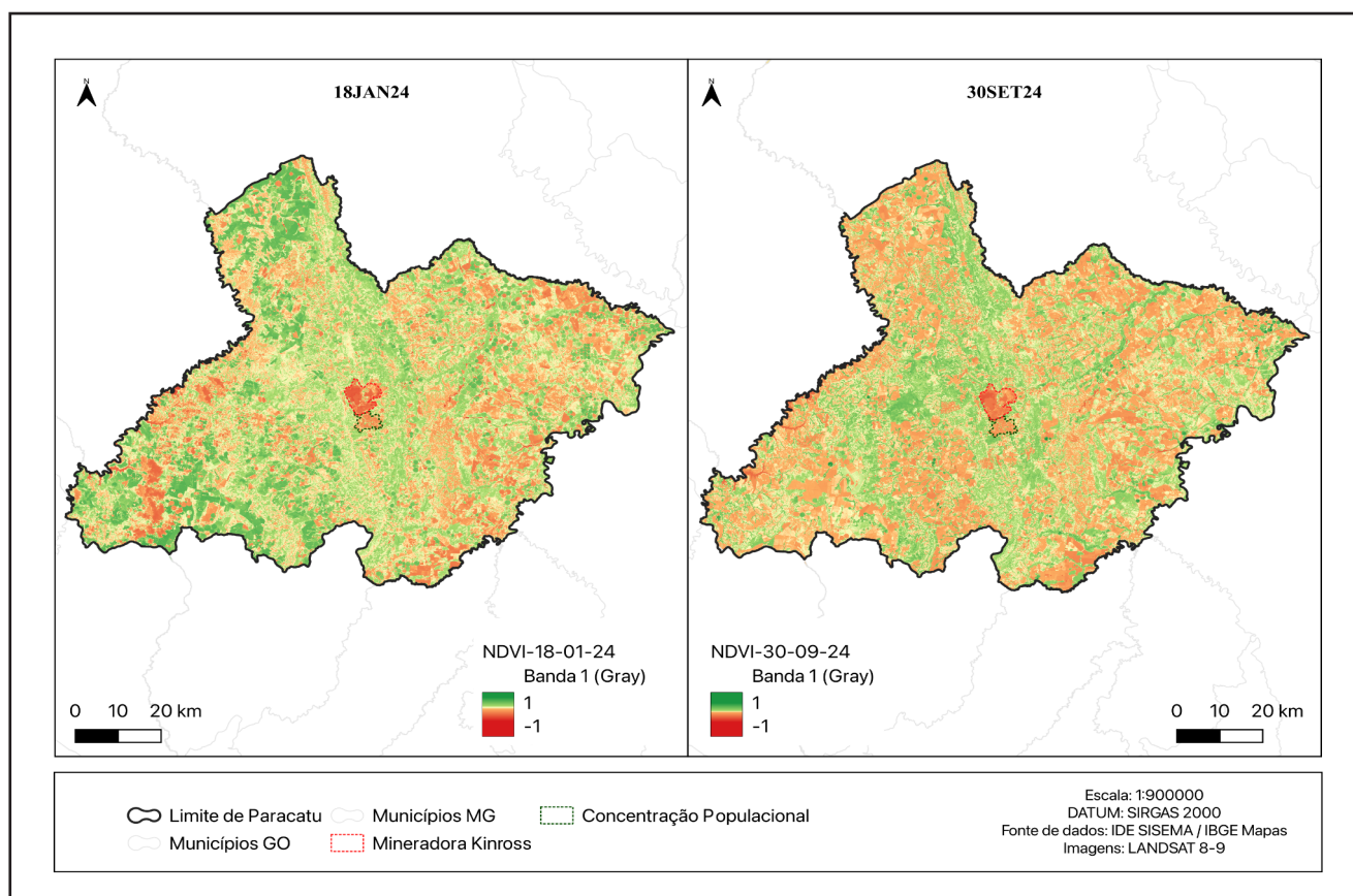
Figura 15. NDVI 2024
