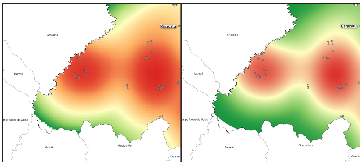
Figura 10. Representação do tamanho do pixel de kernel .
