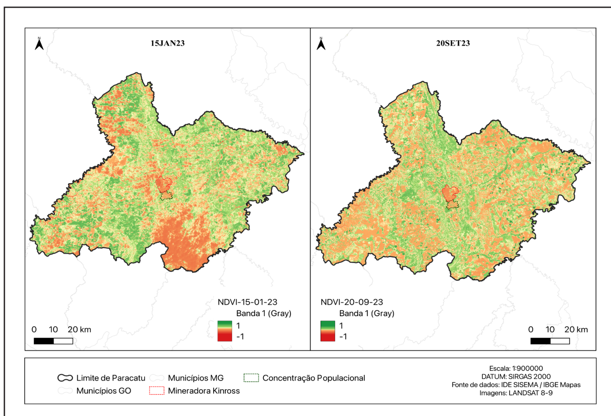
Figura 14. NDVI 2023
