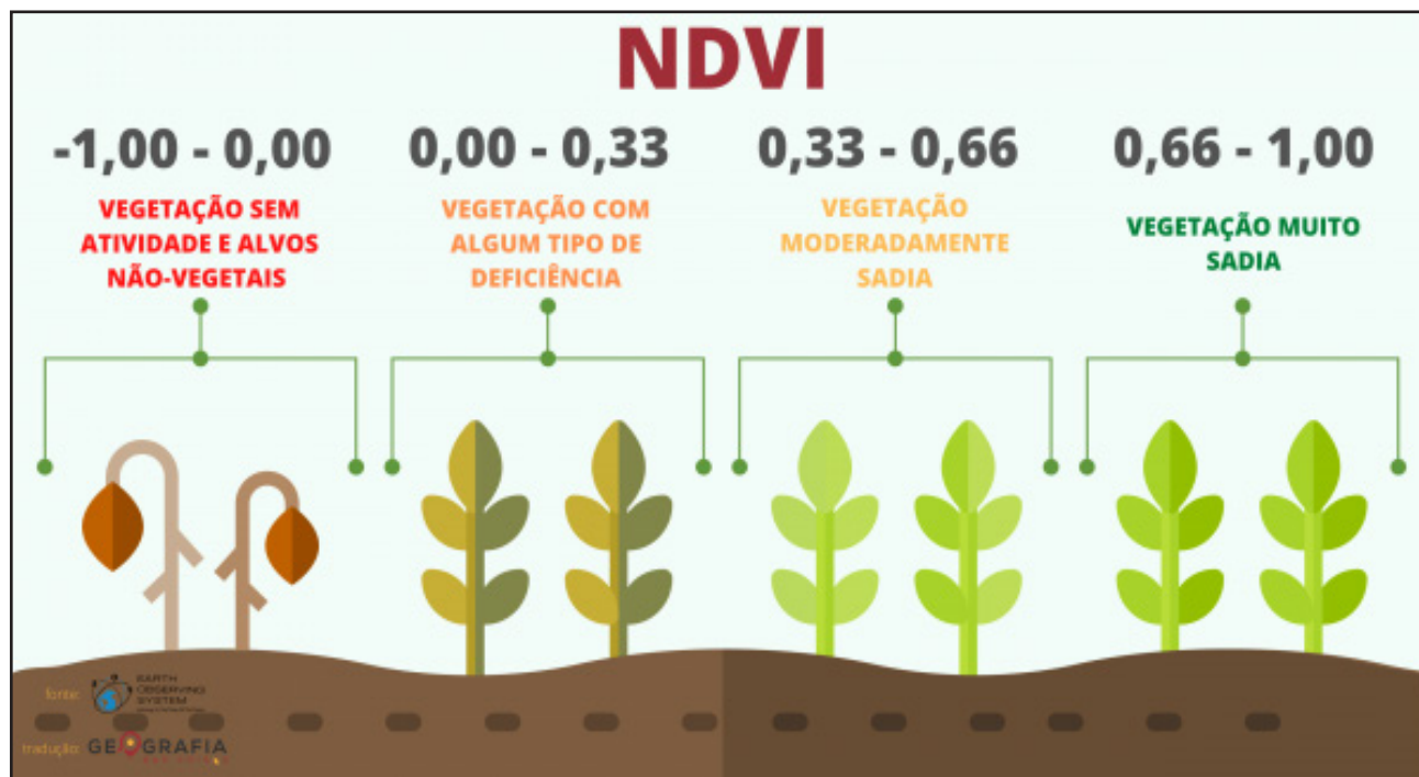
Figura 4. Relação entre o NDVI e a saúde da vegetação
