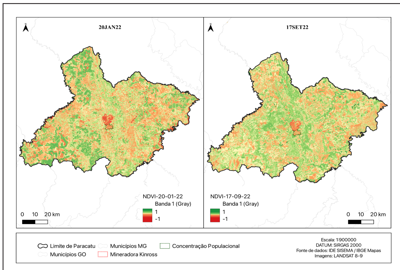
Figura 13. NDVI 2022
