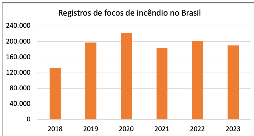
Figura 1. Número de focos de incêndio de 2018 a 2023
