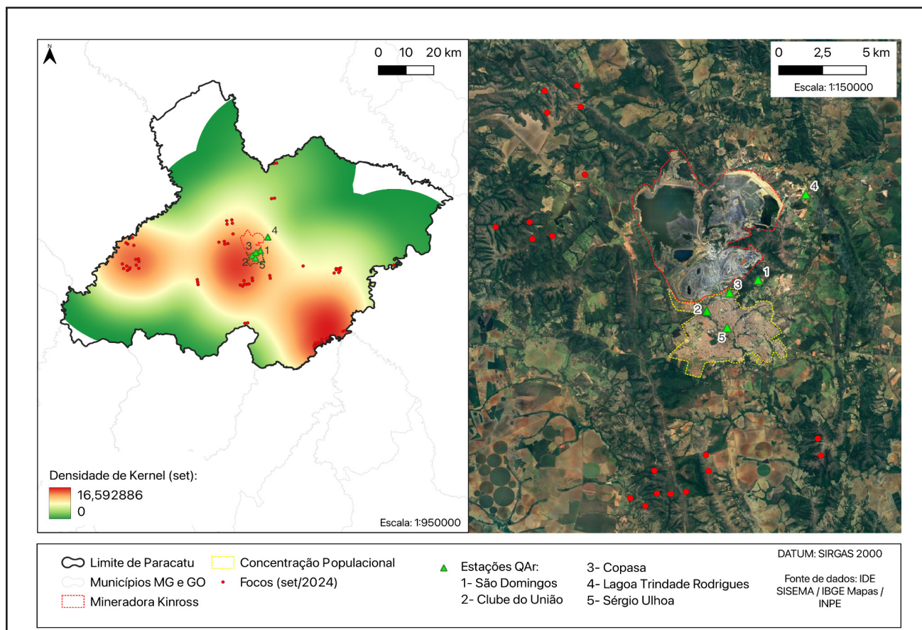
Figura 24. Estimador de Kernel, focos de incêndio e estações de QAr.
