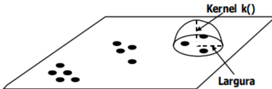
Figura 9. Método de Kernel.
