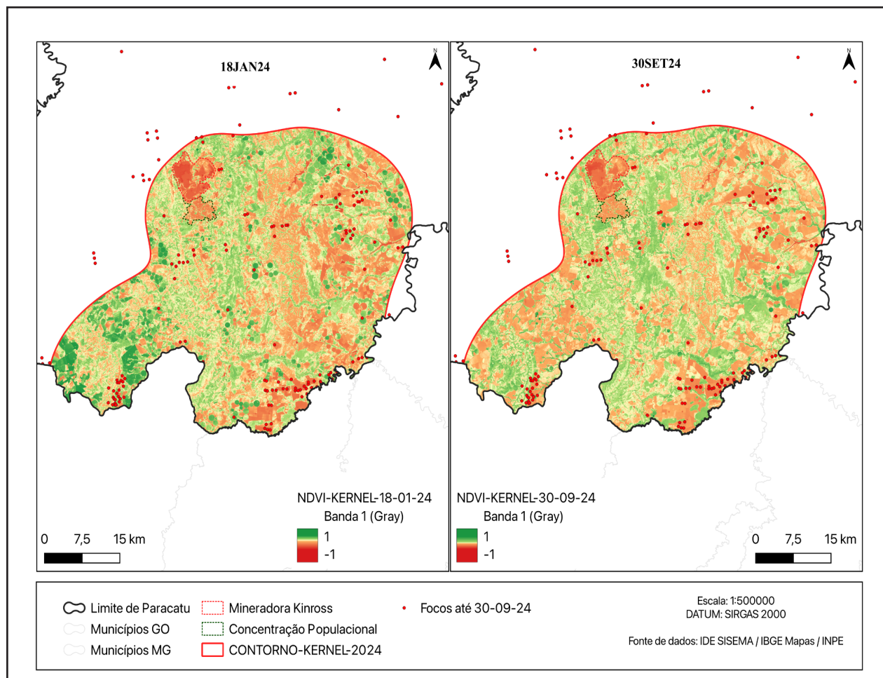
Figura 21. Área de maior densidade de Kernel e NDVI (2024)
