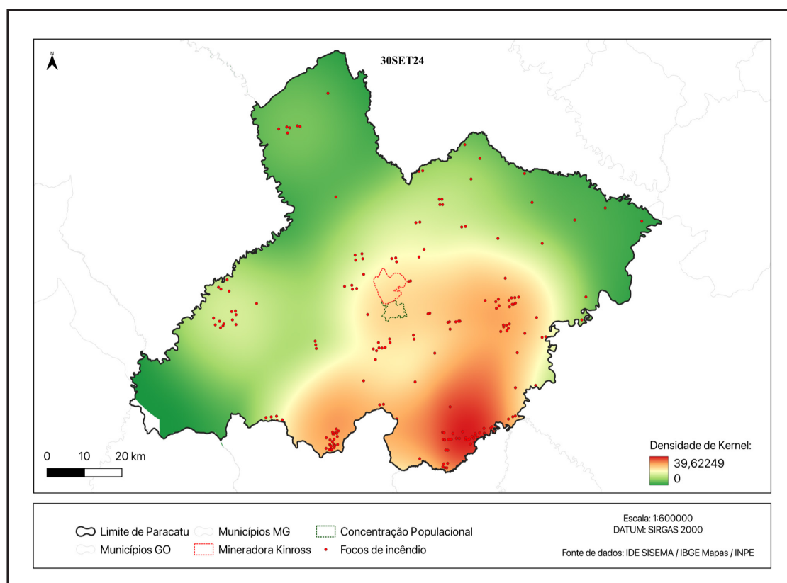
Figura 20. Estimador de Kernel para os focos de incêndio até 30SET24
