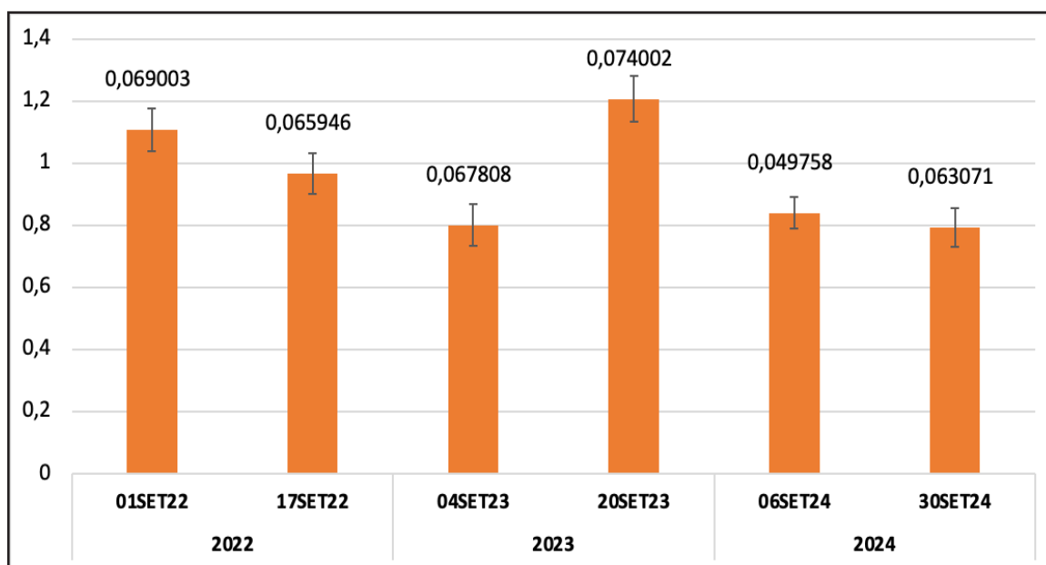
Figura 12. Variação do NDVI e desvio padrão para os dados de setembro
