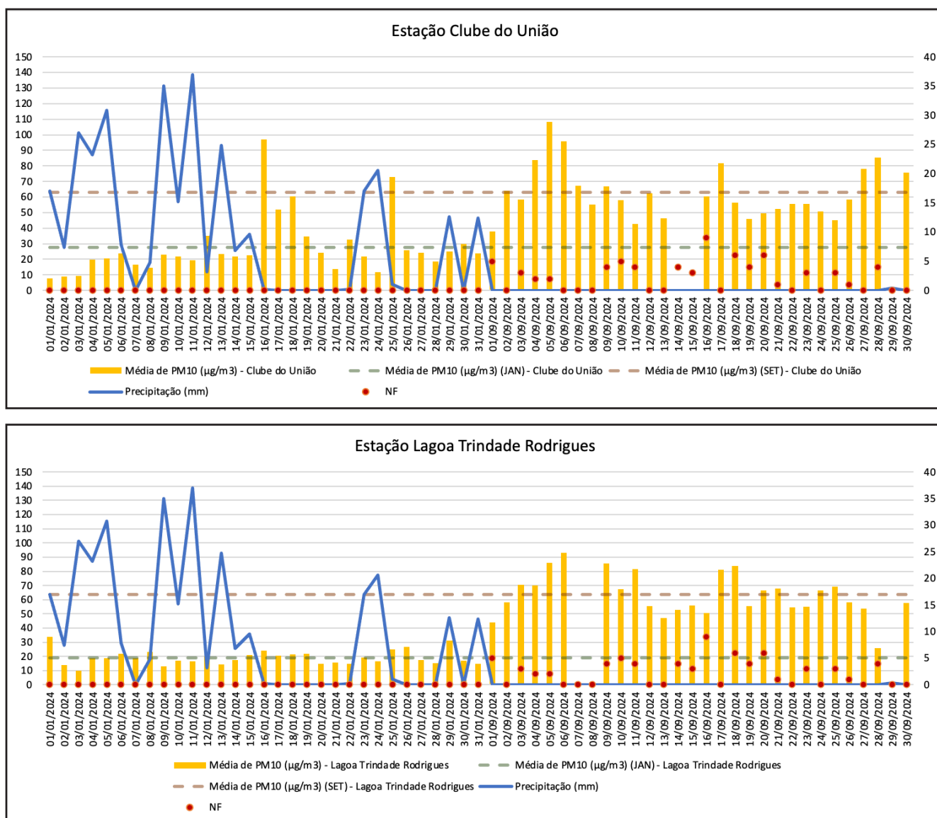
Figura 23. NF, PM_{10} e precipitação para as estações Clube do União (a), Lagoa Trindade Rodrigues (b) e Sérgio Ulhoa (c).
