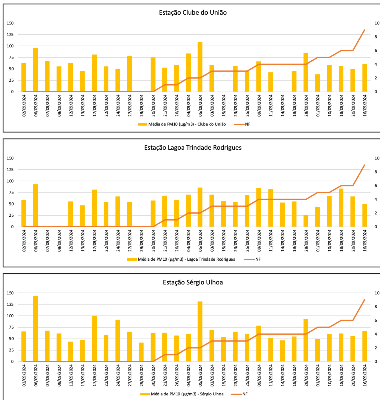
Figura 25. NF e PM 10 para as estações Clube do União (a), Lagoa Trindade Rodrigues (b) e Sérgio Ulhoa (c).
