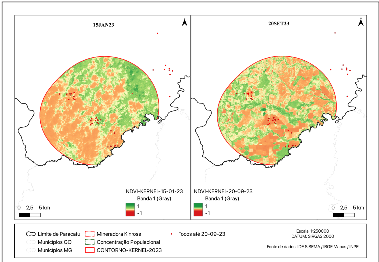
Figura 19. Área de maior densidade de Kernel e NDVI (2023)
