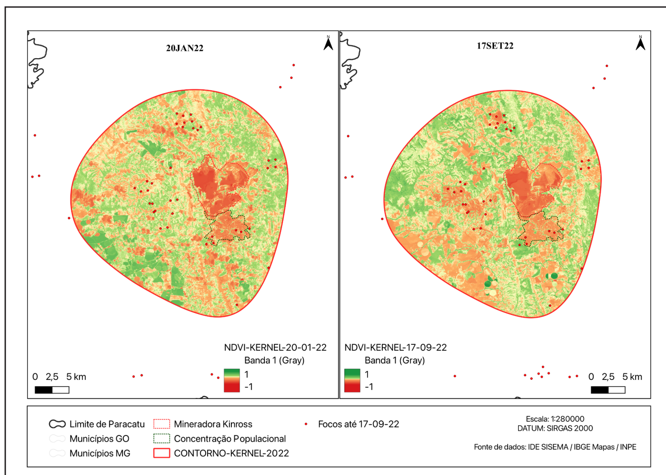
Figura 17. Área de maior densidade de Kernel e NDVI (2022)
