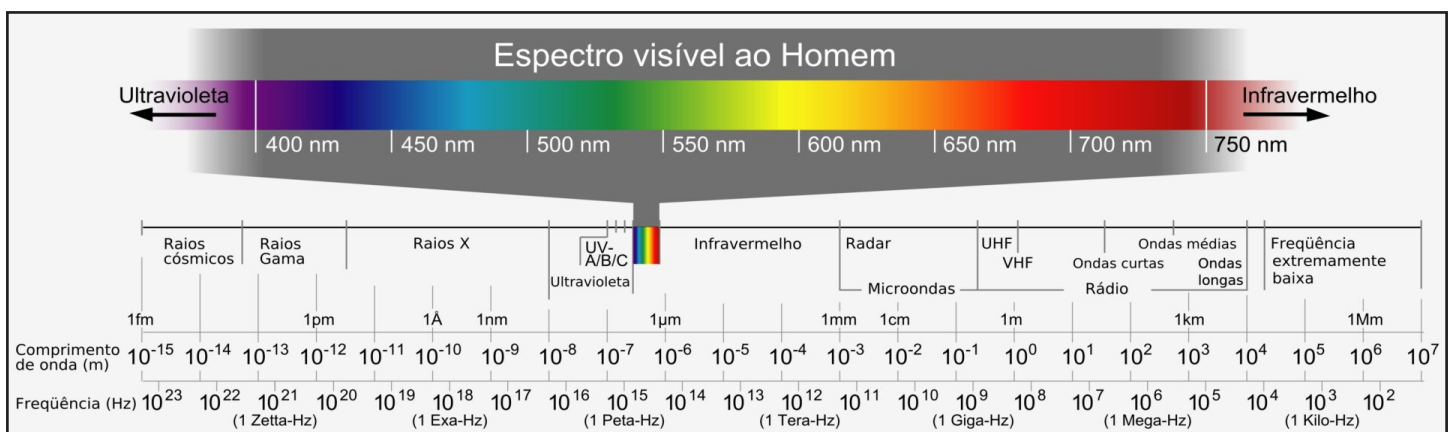
Figura 3. Espectro eletromagnético.
