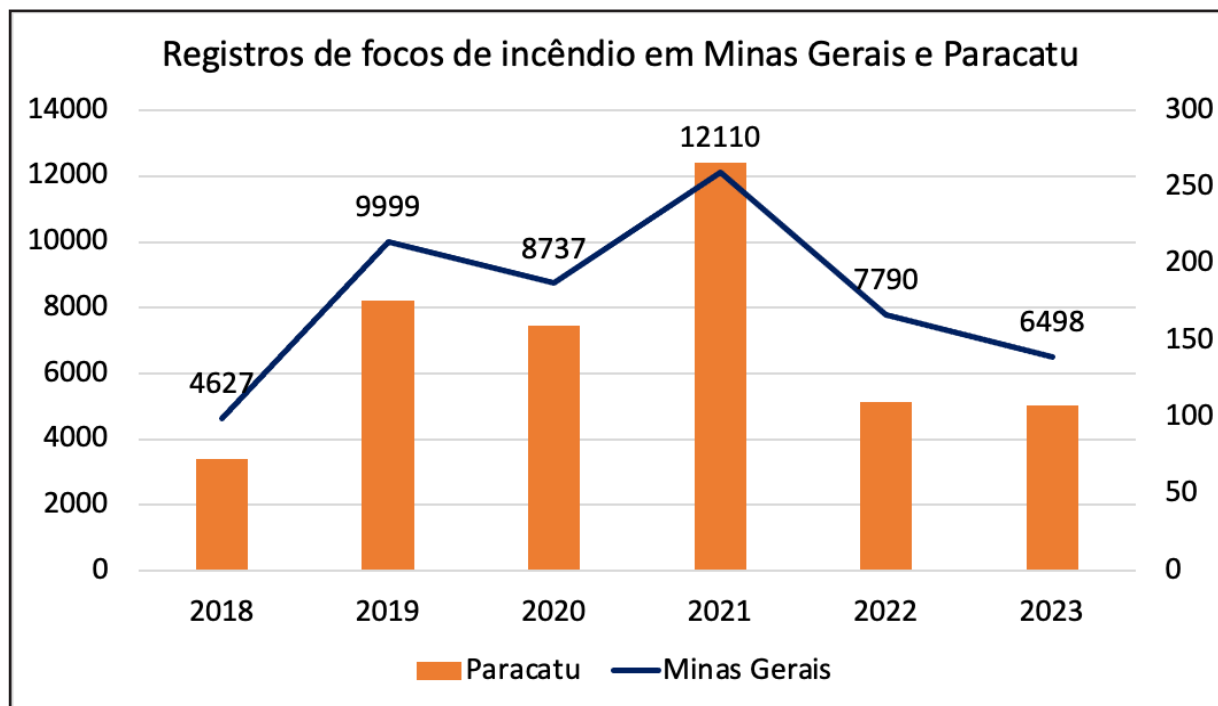
Figura 6. Número de focos de incêndio de 2018 a 2023 para Minas Gerais e Paracatu
